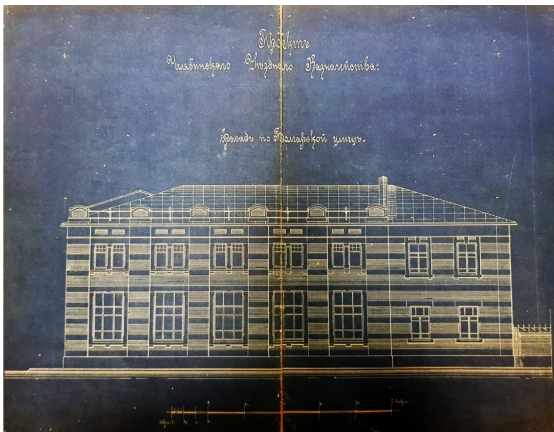
Рис. 8. Проект здания Челябинского уездного казначейства. 1909. Южный фасад. Источник: Архив Отделение по Челябинской области Уральского главного управления Центрального банка РФ.
