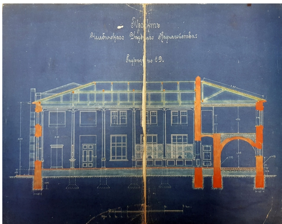
Рис. 5. Проект здания Челябинского уездного казначейства. 1909. Разрез. Источник: Архив Отделение по Челябинской области Уральского главного управления Центрального банка РФ.
