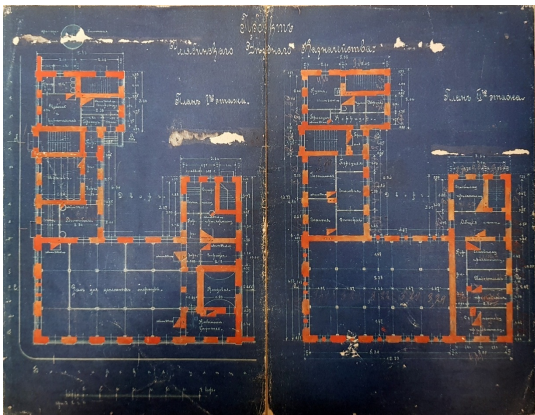
Рис. 6. Проект здания Челябинского уездного казначейства. 1909. Планы этажей. Источник: Архив Отделение по Челябинской области Уральского главного управления Центрального банка РФ.
